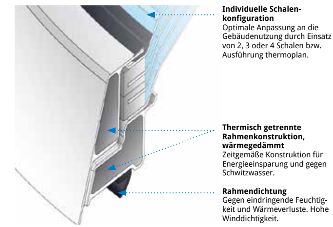
Lichtkuppel essertop® rund
