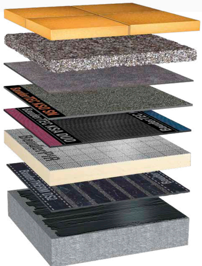
Systemaufbau-Beispiel: BauderPIR FA-TE
